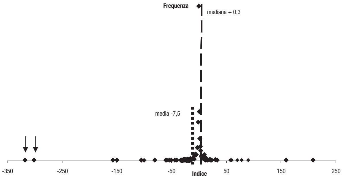
DISTRIBUZIONE STATISTICA DI UN INDICE GENERICO
